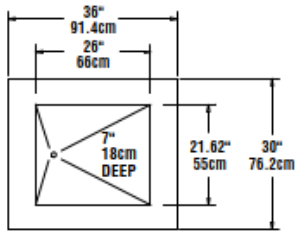
PLAN VIEW KCI-36/ KCI-36-NU
