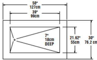
PLAN VIEW KCI-50/ KCI-50-NU
