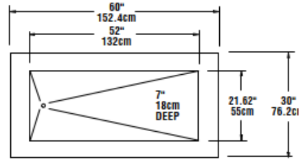
PLAN VIEW KCI-60/ KCI-60-NU
