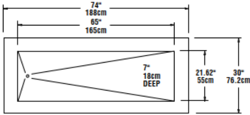
PLAN VIEW KCI-74/ KCI-74-NU
