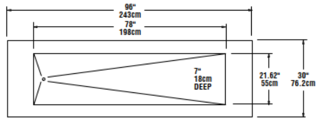
PLAN VIEW KCI-96/ KCI-96-NU
