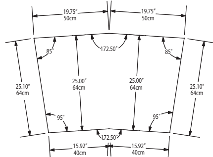
N8044-R Cutout Dimensions
