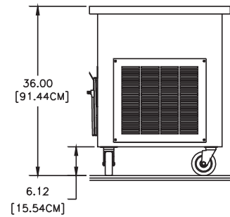
TYP END VIEW
